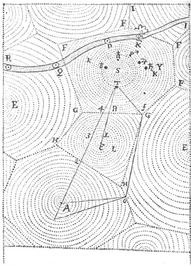
FIGURA 47. — La cosmología de los torbellinos de Descartes, reproducida de su obra Le monde ou le traité de la lumière . Los puntos S, E, A y ε son los centros de los torbellinos. Los rápidos movimientos en torbellino de los corpúsculos centrales los convierten en luminosos, por lo que actúan a modo de estrellas. Los diversos círculos punteados, que no es necesario que conformen circunferencias perfectas, representan los caminos descritos por las corrientes corpusculares, eternamente en rotación, que constituyen el torbellino. Los puntos negros situados alrededor del centro S del torbellino son los planetas, que se ven arrastrados a lo largo de sus respectivas órbitas por el movimiento de los torbellinos. El cuerpo C, situado en la parte superior del diagrama, es un cometa que atraviesa los diferentes torbellinos en una región en la que su movimiento es demasiado lento para constreñirlo sobre una órbita circular continua. El espacio exterior al diagrama está asimismo lleno de torbellinos y cada uno de ellos, al menos potencialmente, representa la localización de un sistema solar en el seno del universo copernicano de Descartes poblado por una infinidad de mundos.
