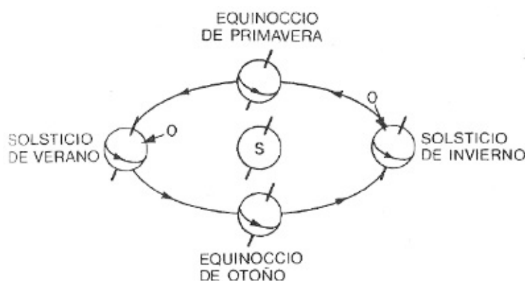
FIGURA 29. — Movimiento anual de la tierra sobre su órbita copernicana. El eje terrestre permanece constantemente paralelo a si mismo o a la recta fija que atraviesa el sol. En consecuencia, un observador O que al mediodía esté situado en latitudes boreales medias ve al sol mucho más alto en el cielo en el solsticio de verano que en el solsticio de invierno.
