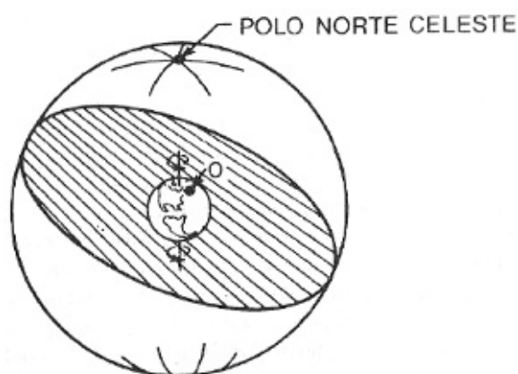
FIGURA 26. — Tierra en rotación situada en el centro de una esfera estelar estacionaria. Comparando este diagrama con el ofrecido en la figura 11, se observará que aquí el plano de horizonte debe girar solidariamente con la tierra para conservar su posición geométrica relativa respecto al observador situado en O.
