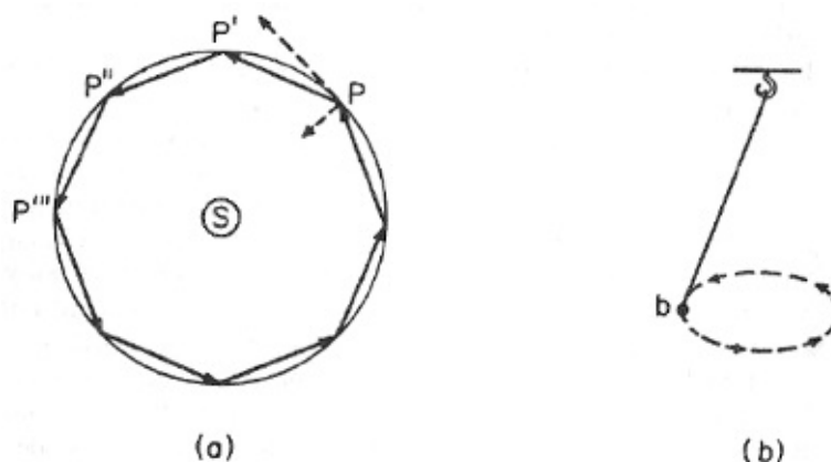
FIGURA 50. — Teoría planetaria de Hooke (a) y su demostración por medio del péndulo cónico (b). En el diagrama (a) el planeta se ve sometido en cada uno de los puntos P , P' , P'' ,... a un impulso instantáneo que lo dirige hacia el sol S . A cada nuevo impulso queda modificada la dirección del movimiento inercial del planeta, y el resultado de la acción de todos ellos es un movimiento a lo largo del perímetro de un polígono. Incrementando el número de puntos en los que el planeta es empujado hacia el centro, crece el número de lados del polígono. En el límite, la acción permanente de una fuerza atractiva central produce una órbita circular. La circularidad de este movimiento puede demostrarse físicamente mediante el aparato representado en el diagrama (b). Si sólo recibe un impulso lateral, el plomo b del péndulo se verá atraído a causa de su propio peso hacia un punto próximo al centro del círculo de trazo discontinuo. Sin embargo, si lo que se comunica al plomo es un impulso en una dirección perpendicular al hilo del que se halla suspendido, su peso le llevará forzosamente a moverse según una curva. Si la intensidad del impulso es la adecuada, el movimiento del plomo tendrá lugar a lo largo de un círculo horizontal o de una órbita alargada muy similar a una elipse.
