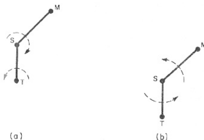
FIGURA 38. — Equivalencia geométrica del sistema de Tycho Brahe (a) y del sistema de Copérnico (b). En (a) el sol S es arrastrado por el brazo rígido TS en su movimiento hacia el este alrededor de la tierra inmóvil T. Simultáneamente, el planeta Marte M se ve arrastrado hacia el oeste alrededor de S a causa de la rotación regular del brazo SM. Puesto que TS gira más deprisa que SM, el movimiento total de Marte está dirigido hacia el este salvo en el breve periodo en que SM se cruza con TS. El diagrama (b) muestra los mismos brazos girando alrededor del sol inmóvil S. Las posiciones relativas de T, S y M son idénticas en ambos esquemas, situación que se mantiene mientras ambos diagramas giran. En particular, nótese que en (b) también debe decrecer el ángulo TSM, tal como sucede en (a), pues TS gira alrededor del sol con velocidad superior a la que lo hace SM.
