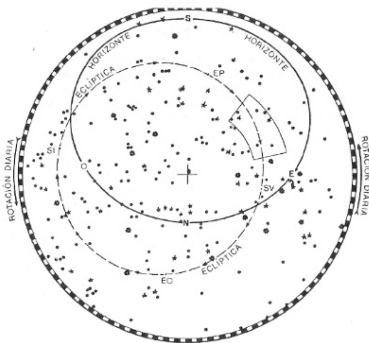
FIGURA 8. — Mapa circumpolar del cielo en el que aparecen las principales estrellas visibles permanentemente para un observador situado alrededor de los 45° de latitud norte. La cruz situada en el centro geométrico del mapa señala la posición del polo celeste.
